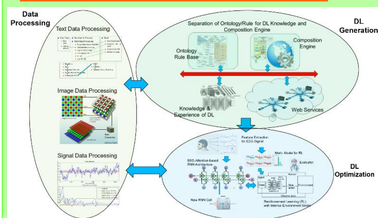
DL生成システム概要
