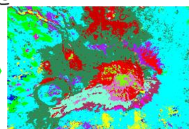
（作成する地質図のイメージ）
