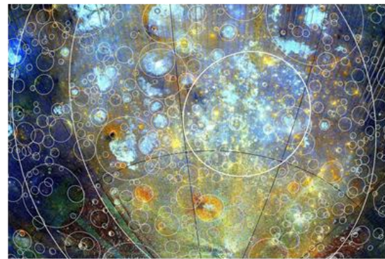
衛星観測データによる地質情報の例 （月周回衛星「かぐや」のデータ）
